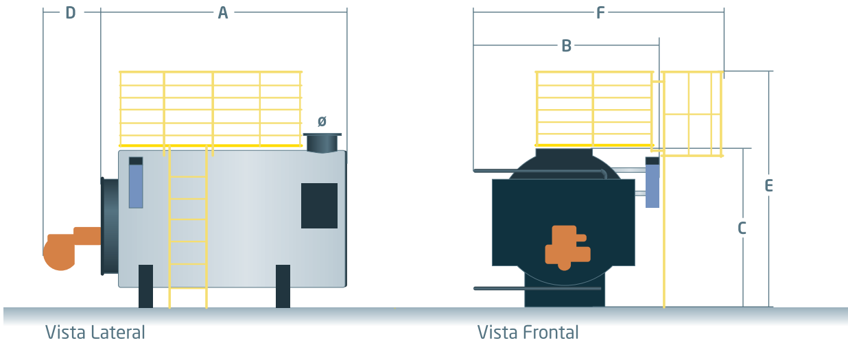
Dimensões CVSHP | 1.000 a 8.000kg/h de vapor
